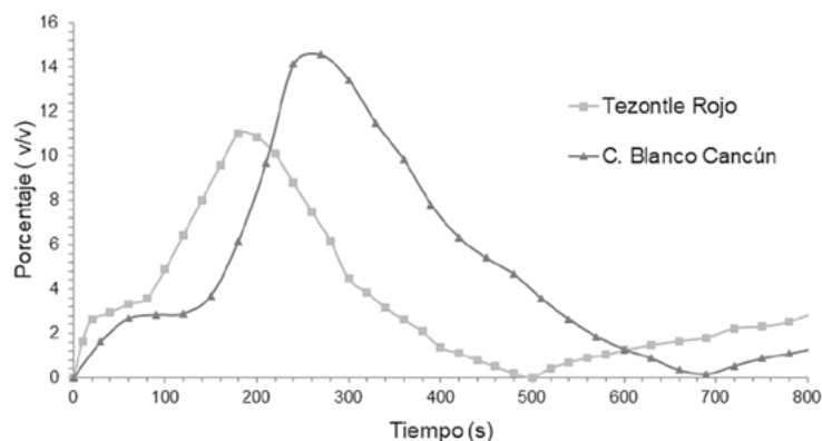
Figura 1. Tiempo de residencia real promedio de la columna de adsorción, a partir de la inyección de azul de bromotimol.
